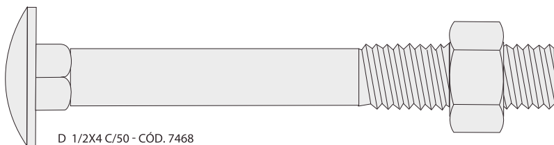
D 1/2x4 C/50 - Cód. 7468
