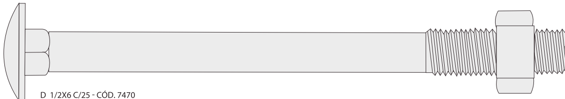
D 1/2x6 C/25 - Cód. 7470
