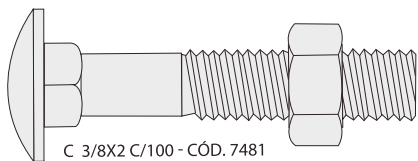
C 3/8x2 C/100 - Cód. 7481
