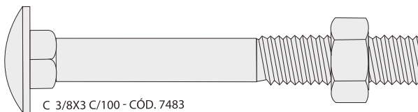
C 3/8x3 C/100 - Cód. 7483
